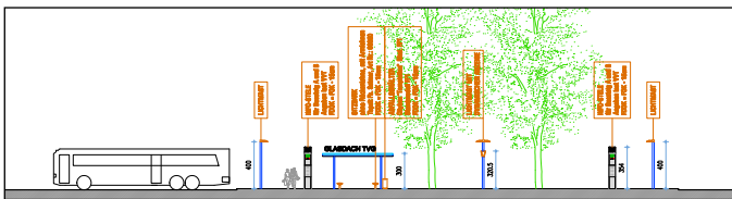
Bussteig in Längsansicht
